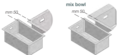
distanza foro incasso cutout spacing
